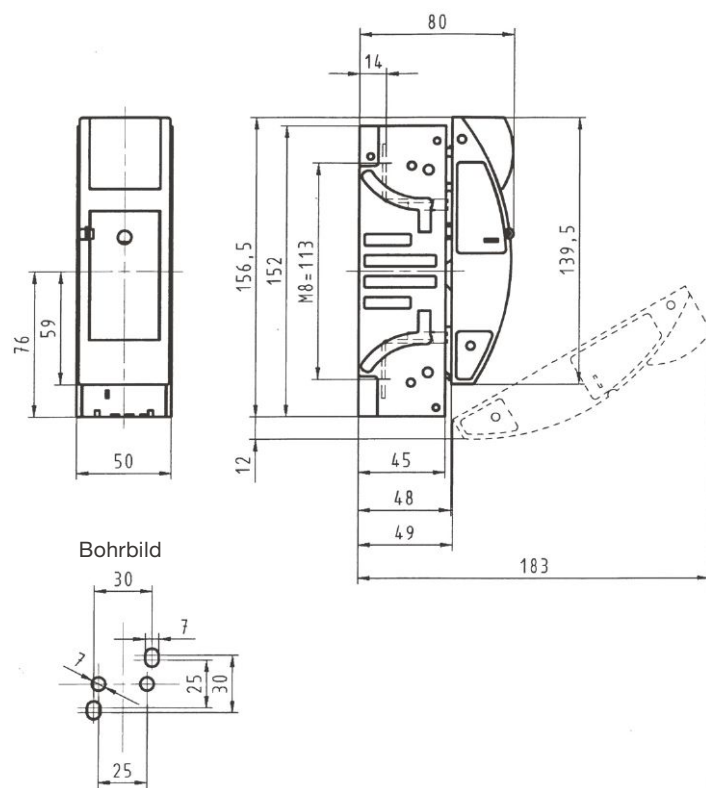
Maßbilder 33136-0010
