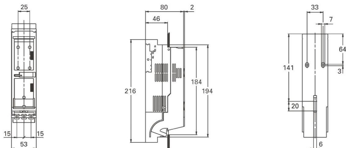
Maßbilder Größe 00
