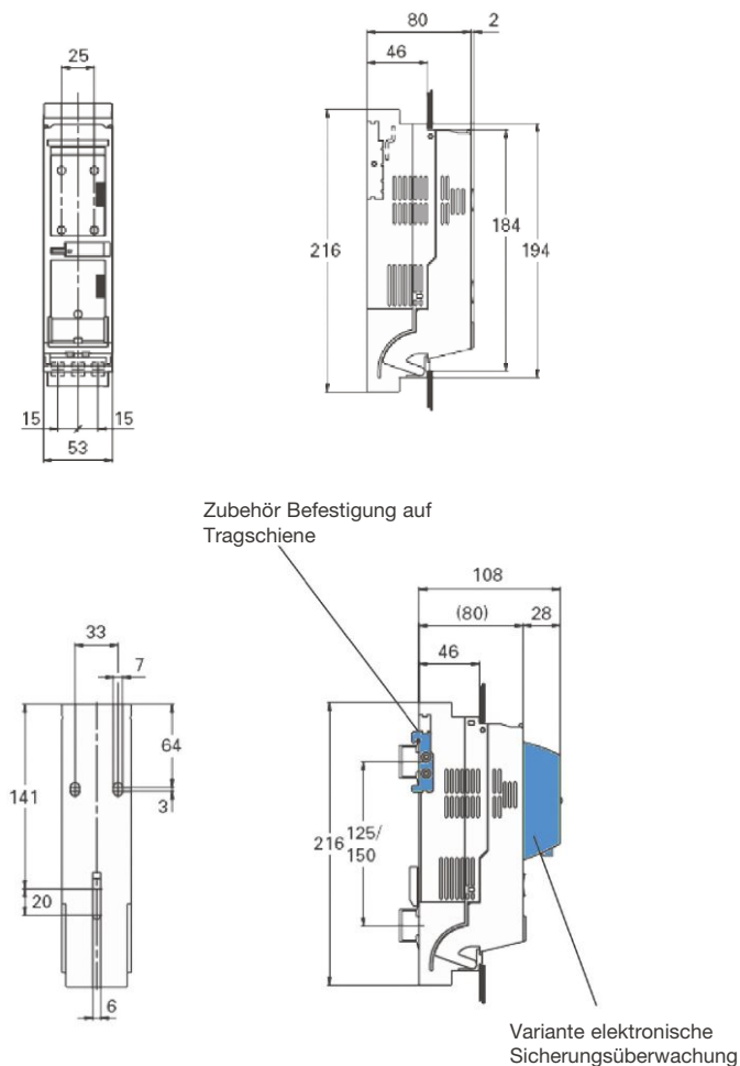
Größe 000, schmale Ausführung
