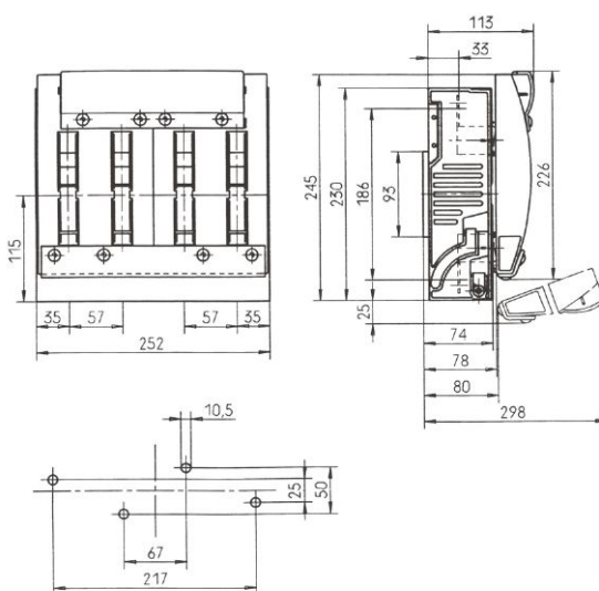
Maßbilder Größe 1, 250 A
