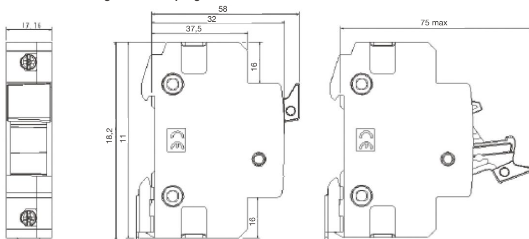
Maße DC-Sicherungs-Trenner 1-polig
