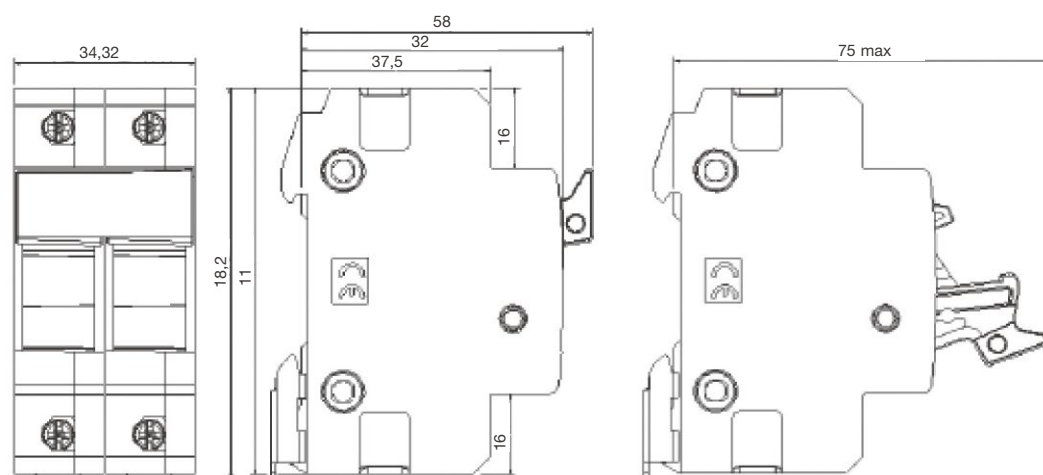
Maße DC-Sicherungs-Trenner 2-polig
