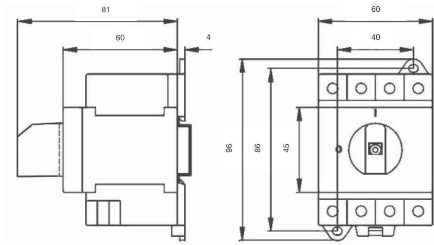
Maße DC-Lastschalter
