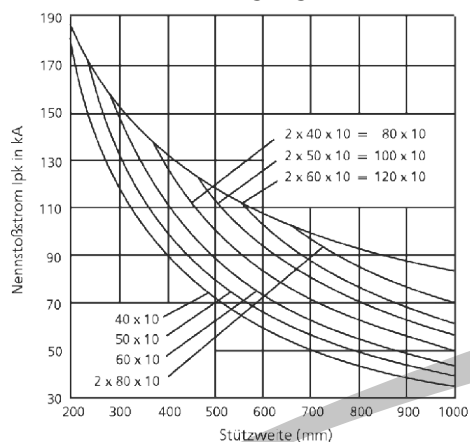
Kurzschlussfestigkeit von SH 100 Vierloch-Befestigung
